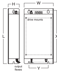
Footprint dimensions
